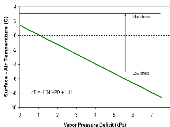
Figura 0.2. Ejemplo de Crop water stress index según el método de Idso, mostrando la distancia relativa de las medidas entre el lower y upper baselines, en función del deficit de presión de vapor. (Idso et al. 1981).
