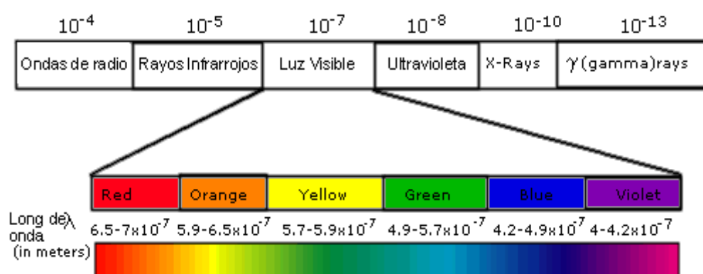
Figura 0.3. Espectro electromagnético
